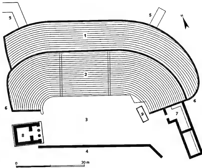
Thorikos, Theater; um 500 v. Chr. (Grundriß). 1 jüngeres kōilon 2 älteres kōilon 3 orchēstra/Spielfläche 4 Terrassenmauer 5 Zugangsrampe 6 Stützmauer 7 Felsenkammern 8 Tempel 9 Altar
